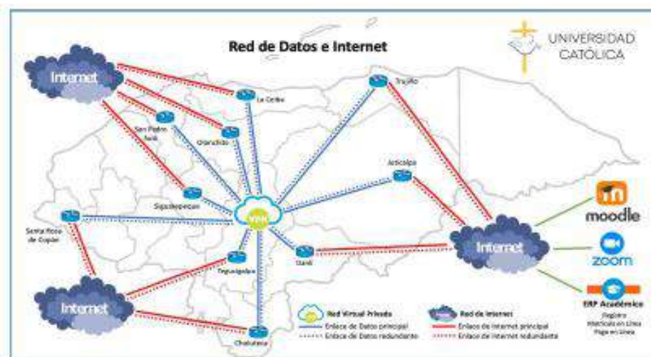
Figura 2. Arquitectura de red y conectividad de la UNICAH, interna e Internet.
